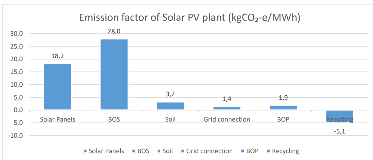
Kuvio 3 Aurinkovoimalan elinkaaren aikaiset päästökertoimet (kgCO 2 -e/MWh)
