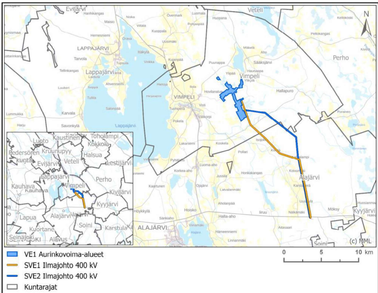
Kuva: Hankealue ja tarkasteltavat sähkönsiirtovaihtoehtot (kuva: Ecobio Oy).
